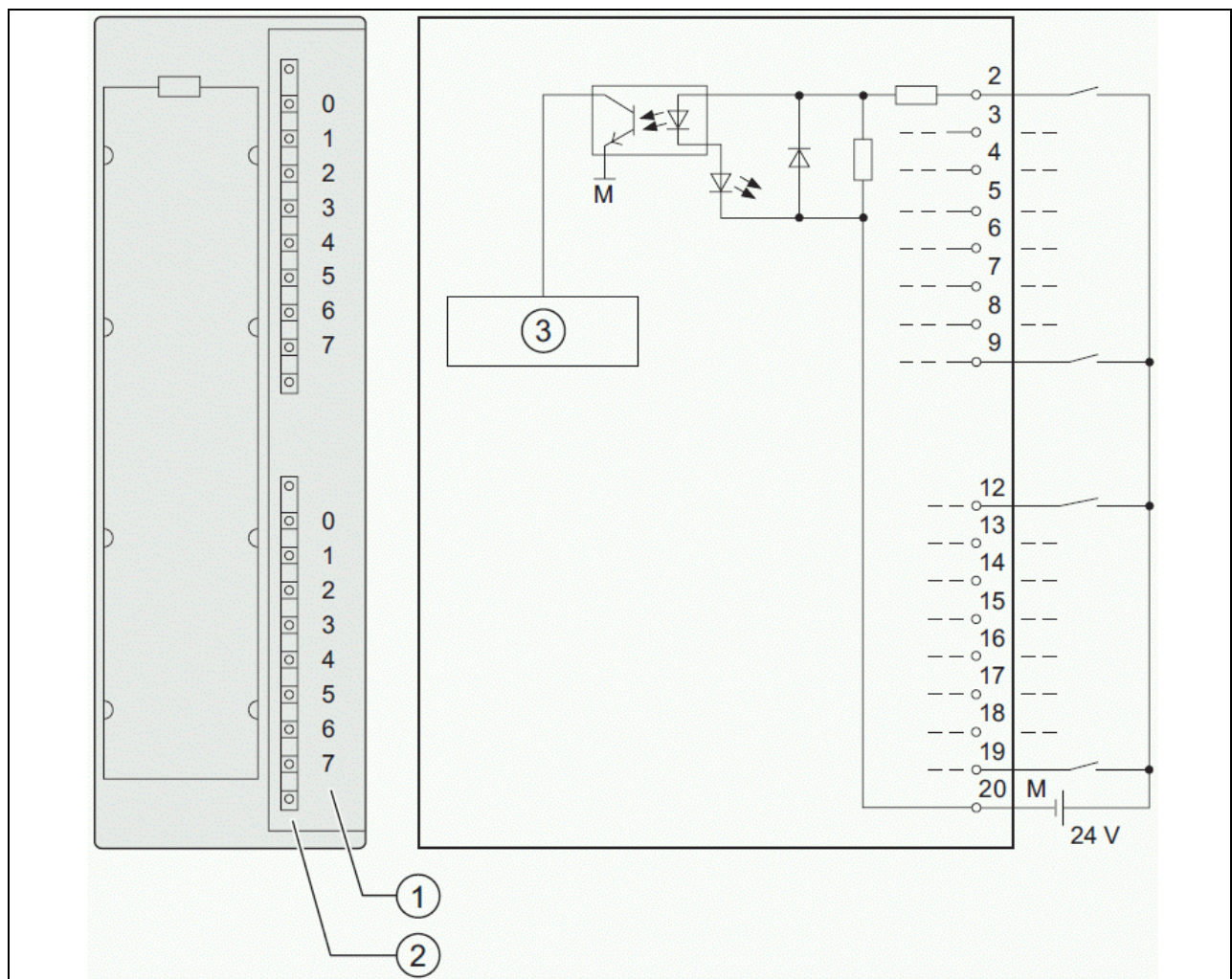
Figura 4.5. Schema bloc a modului S7 321 si schema de cablare la borne a semnalelor de tensiune
