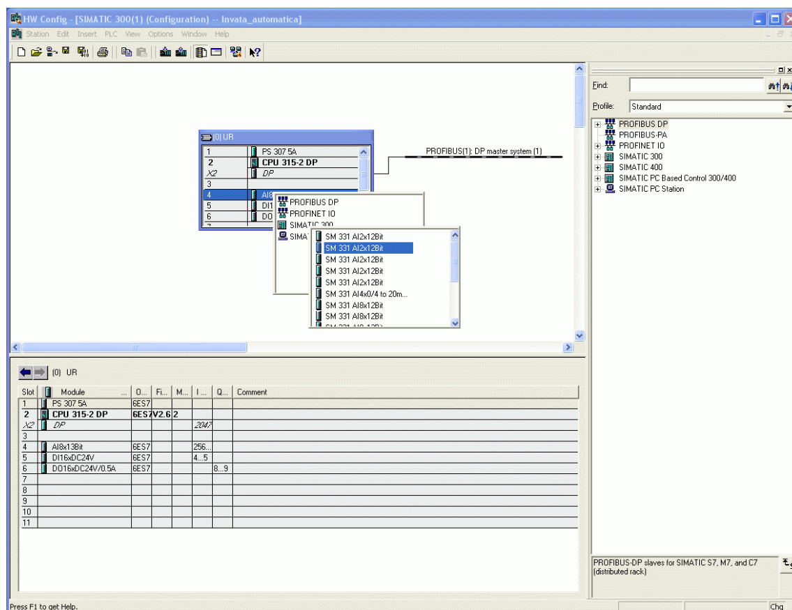
Figura 5.19. Selectia modulului nou SM 331 AI2x12bit
